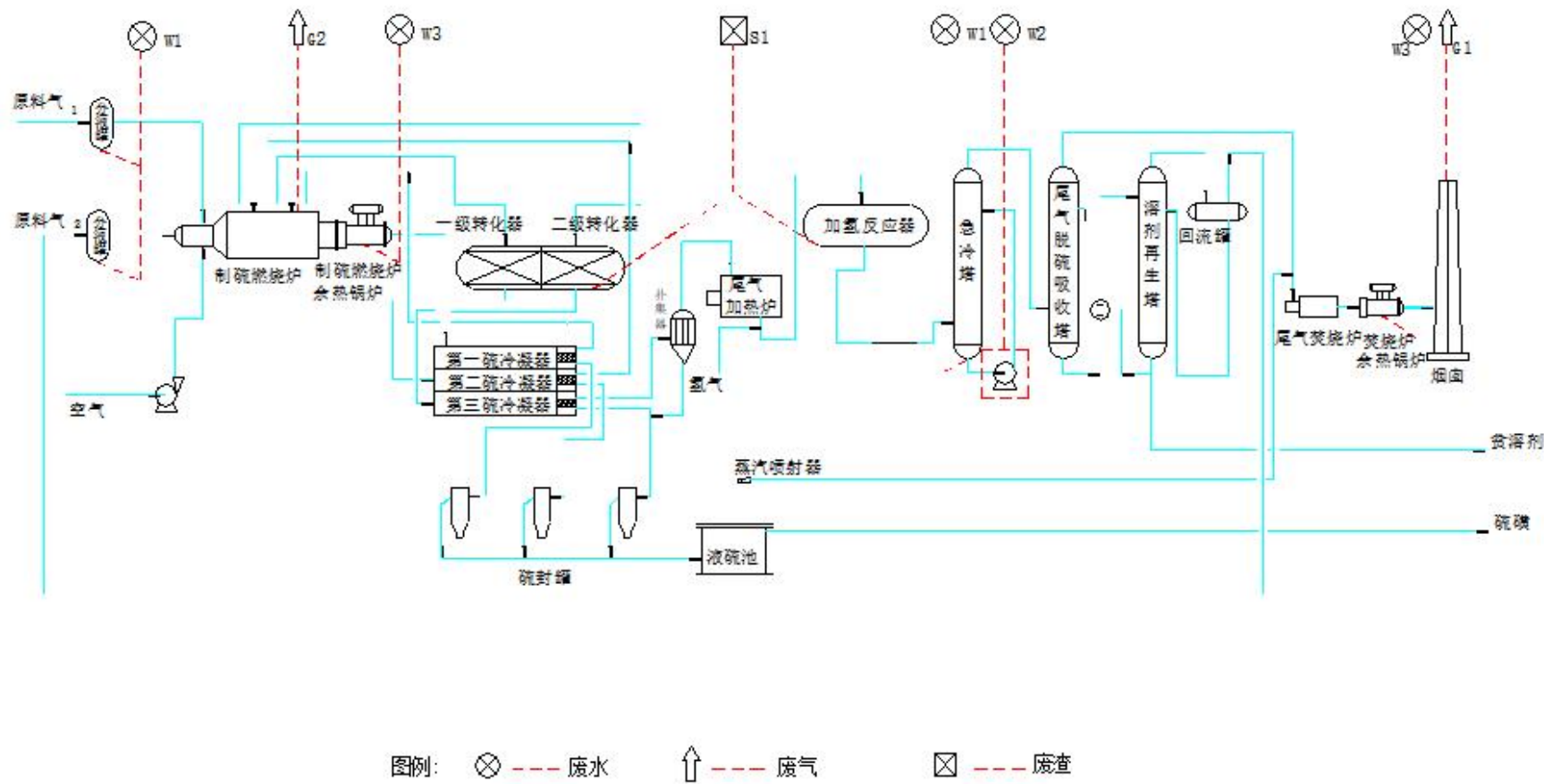
图 4.4-10 制硫装置工艺流程和污染源示意图
