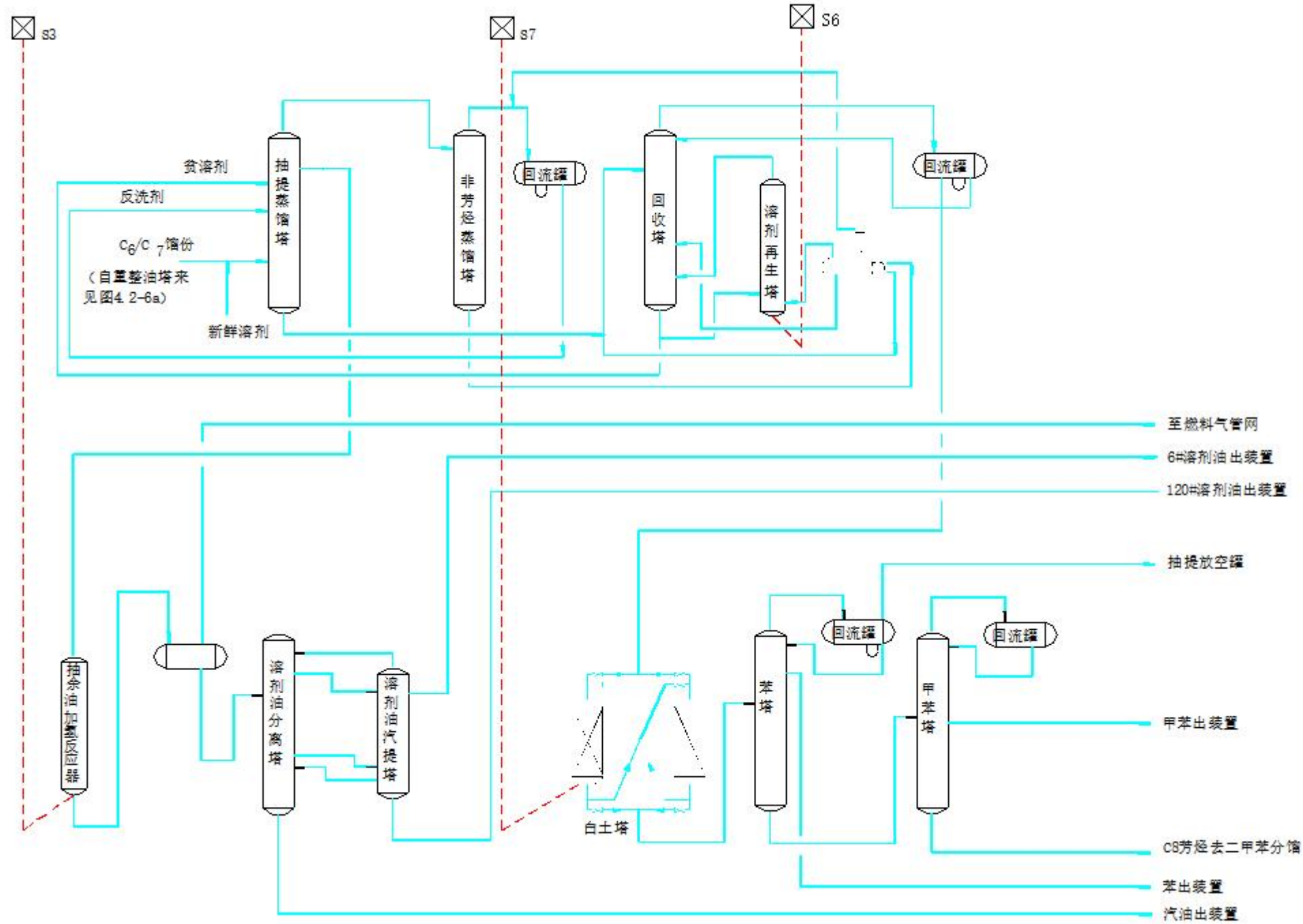
图 4.4-8b 重新抽提装置工艺流程和污染源分布示意图（二）
