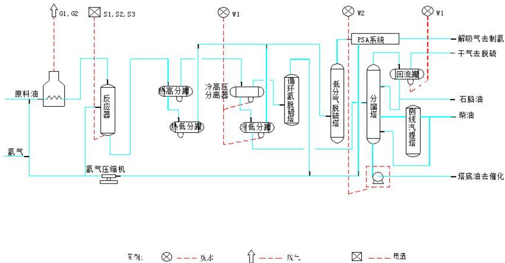
图 4.4-4 蜡油加氢处理装置工艺流程和污染源示意图
