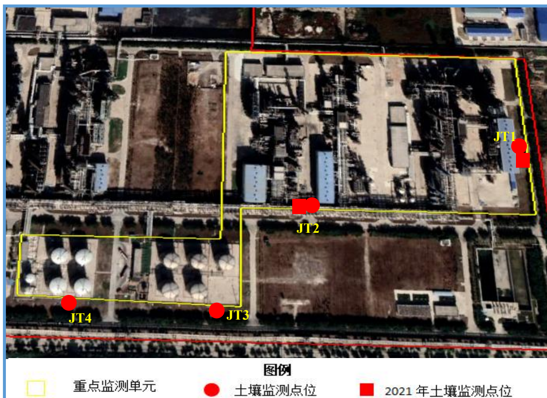
图 6.2-10 渣油加氢装置、蜡油加氢装置、连续重整装置区、403 单元、404 单元区土壤采样点位布置图
