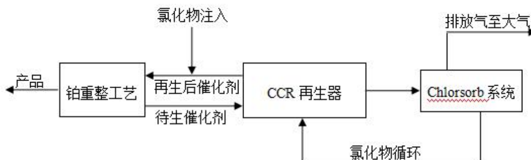
图 4.4-7 催化剂再生工艺流程图
