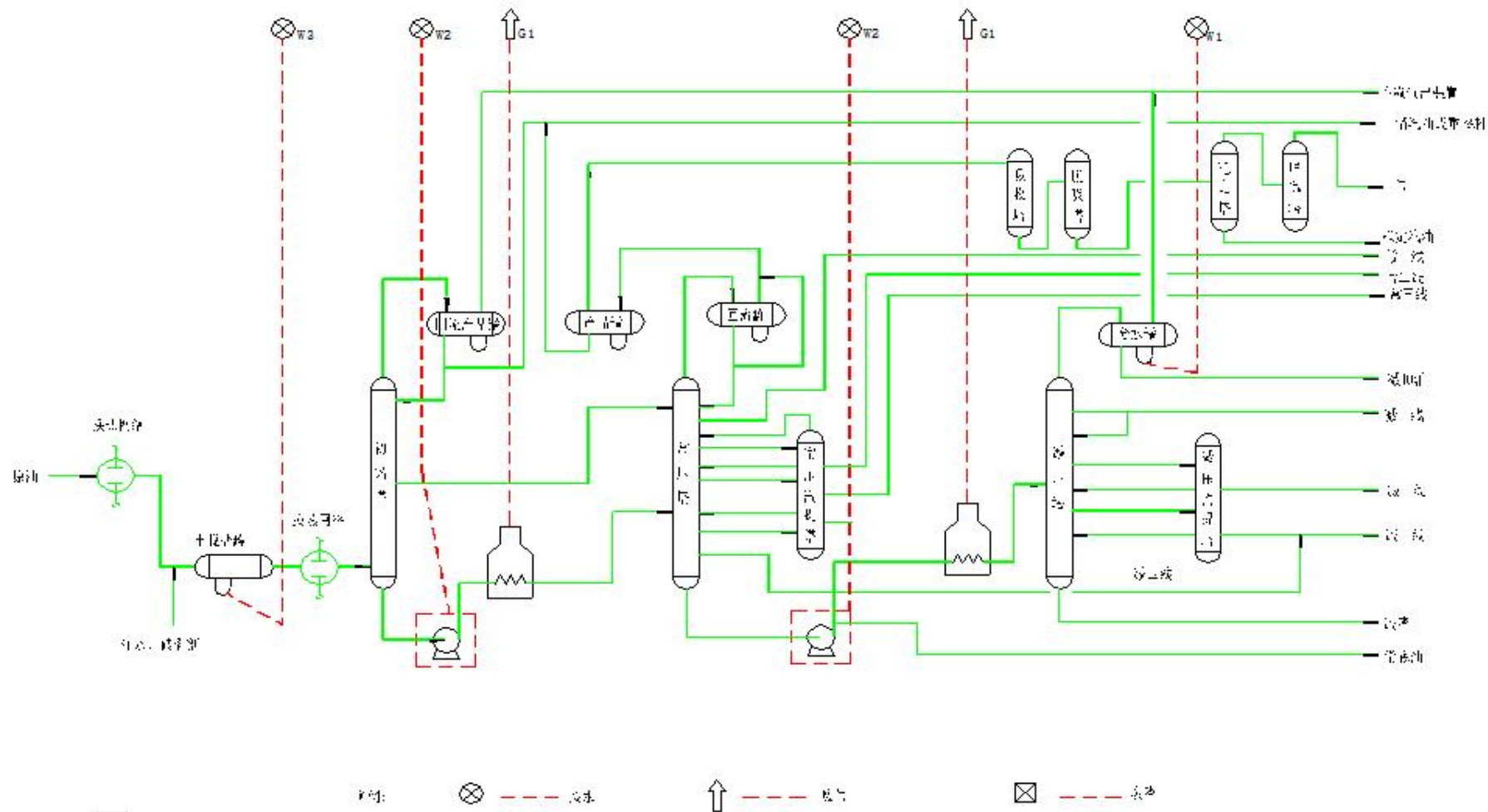
图 4.4-2 常减压装置工艺流程和污染源分布示意图
