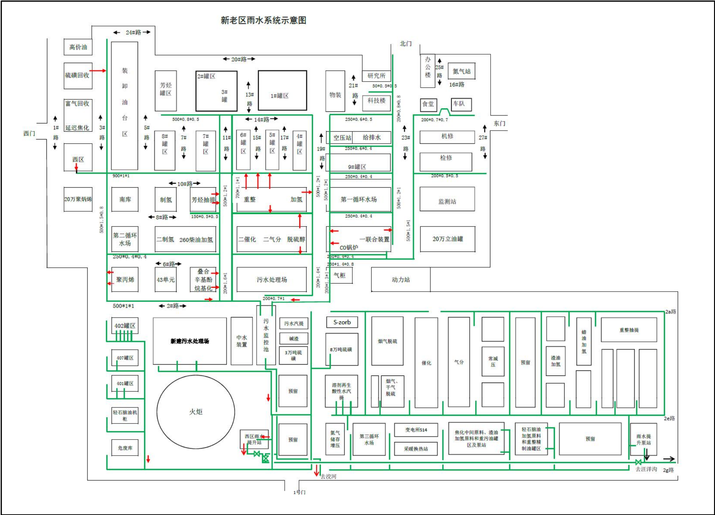
图 4.2-2 地块雨水排放管网图
