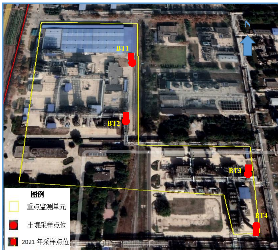
图 6.2-2 聚丙烯、烷基化装置区土壤采样点位布置图
