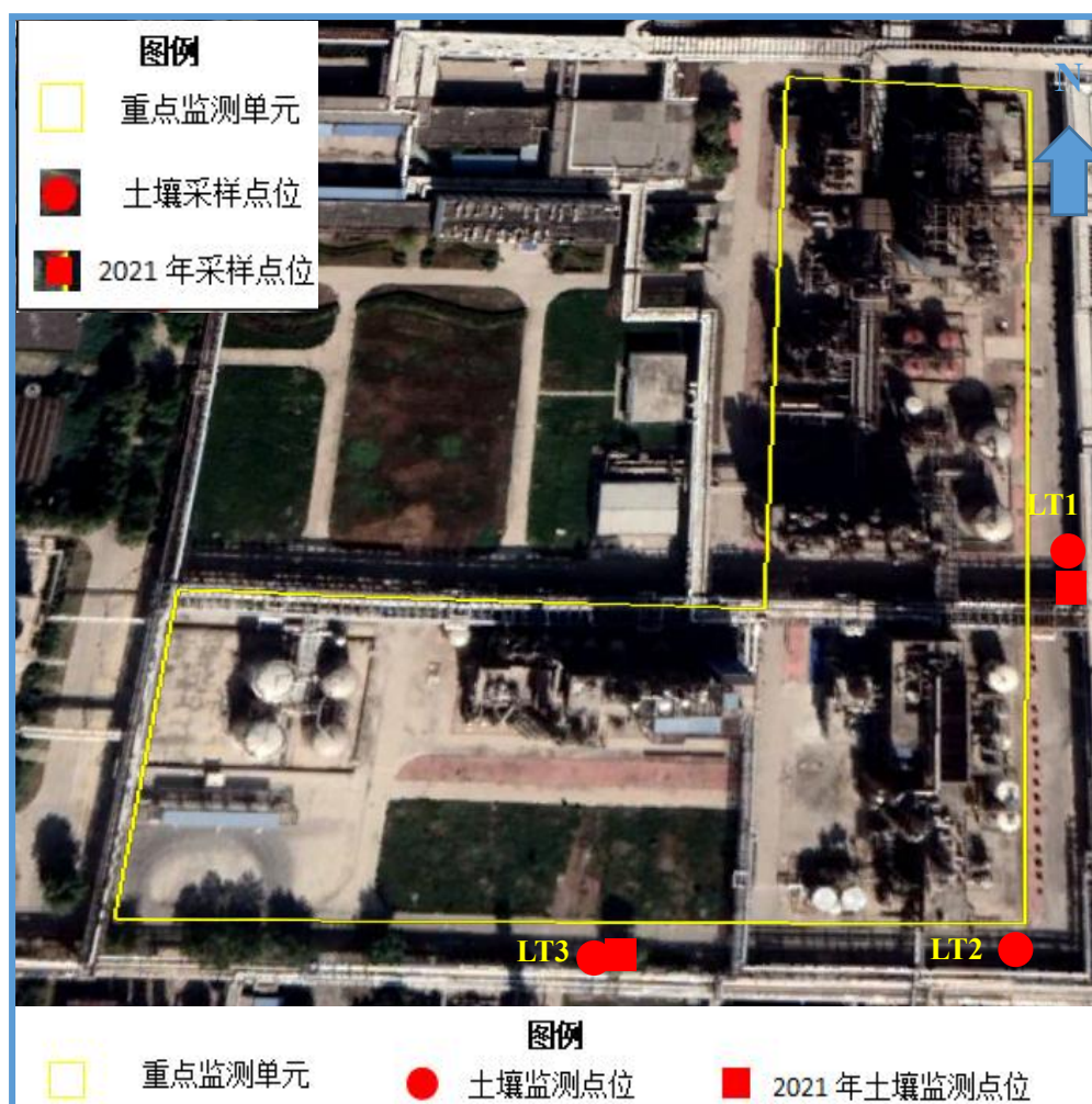
图 6.2-12 己内酰胺装置、氨肟化装置区土壤采样点位布置图
