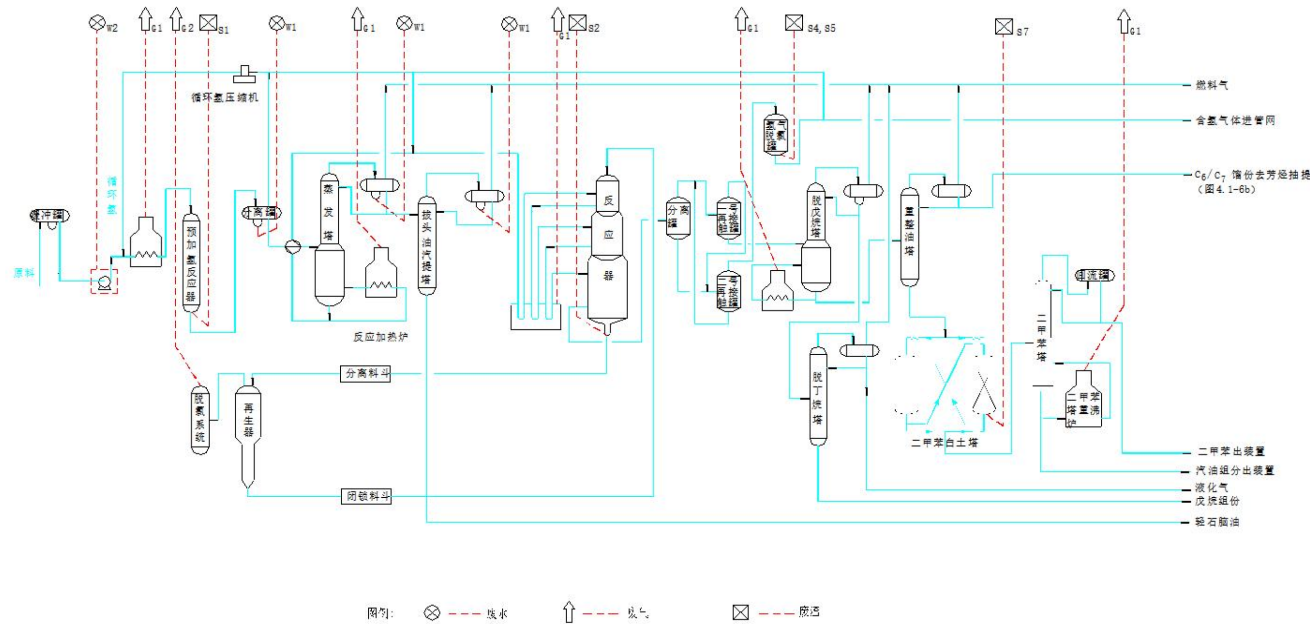
图 4.4-8a 重新抽提装置工艺流程和污染源分布示意图（一）
