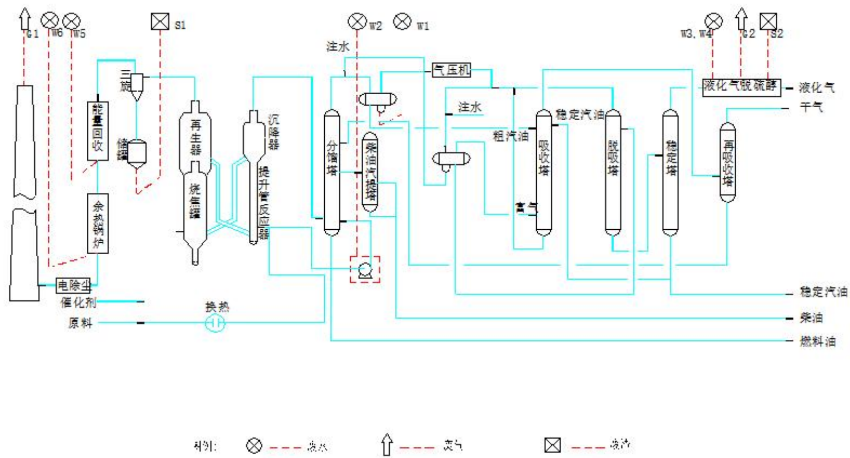
图 4.4-6 催化裂化装置工艺流程和污染源分布示意图
