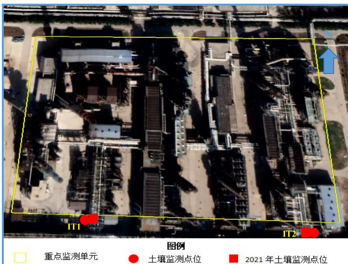
图 6.2-9 2#常减压装置区土壤采样点位布置图
