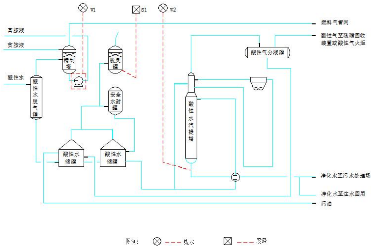
图 4.4-11 酸性水汽提装置工艺流程和污染源示意图
