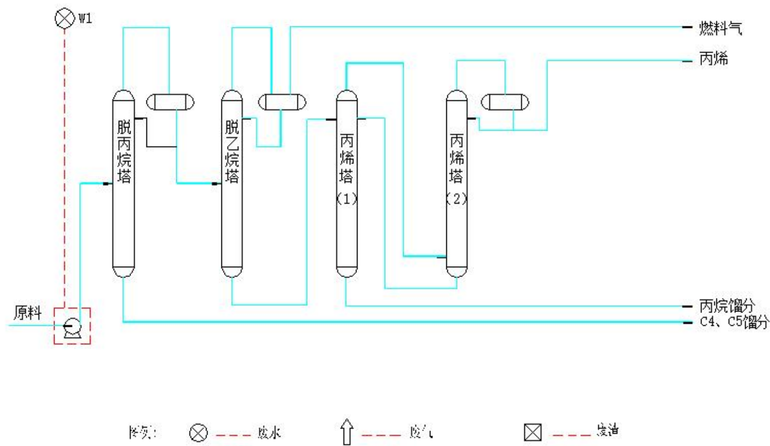
图 4.4-9 气体分馏装置工艺流程和污染源分布示意图
