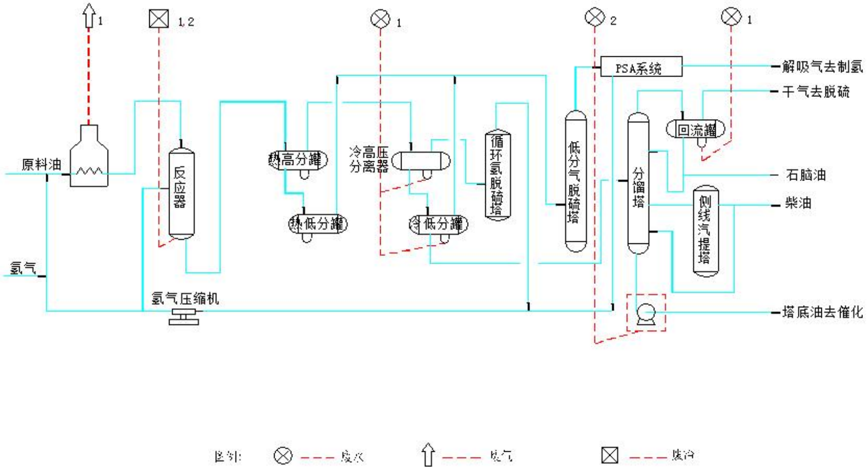
图 4.4-5 催化原料加氢处理装置工艺流程和污染源示意图
