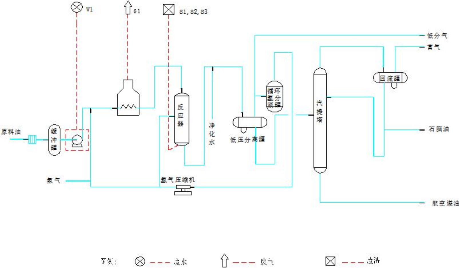
图 4.4-12 航煤加氢装置工艺流程和污染源示意图
